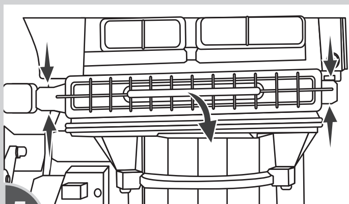
5 PRESIONAR PESTAÑAS Y RETIRAR CUBIERTA
