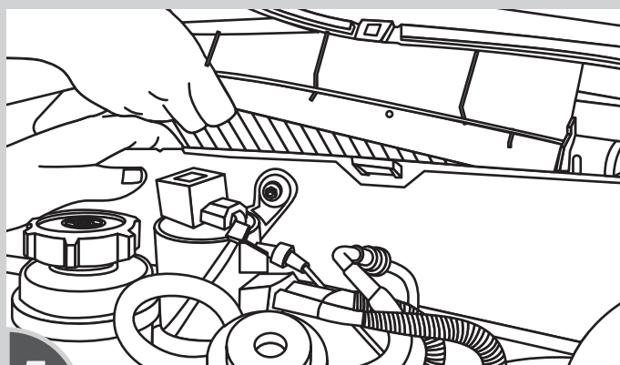
5 LEVANTAR CUBIERTA Y REMOVER FILTRO USADO
