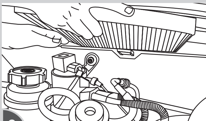
6 INSERTAR FILTRO CON ALAS CERRADAS HACIA ARRIBA
