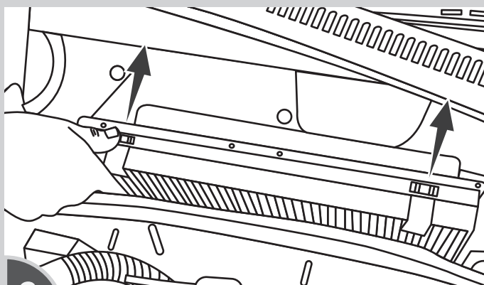
6 RETIRAR FILTRO DE LA BANDEJA Y CAMBIAR
